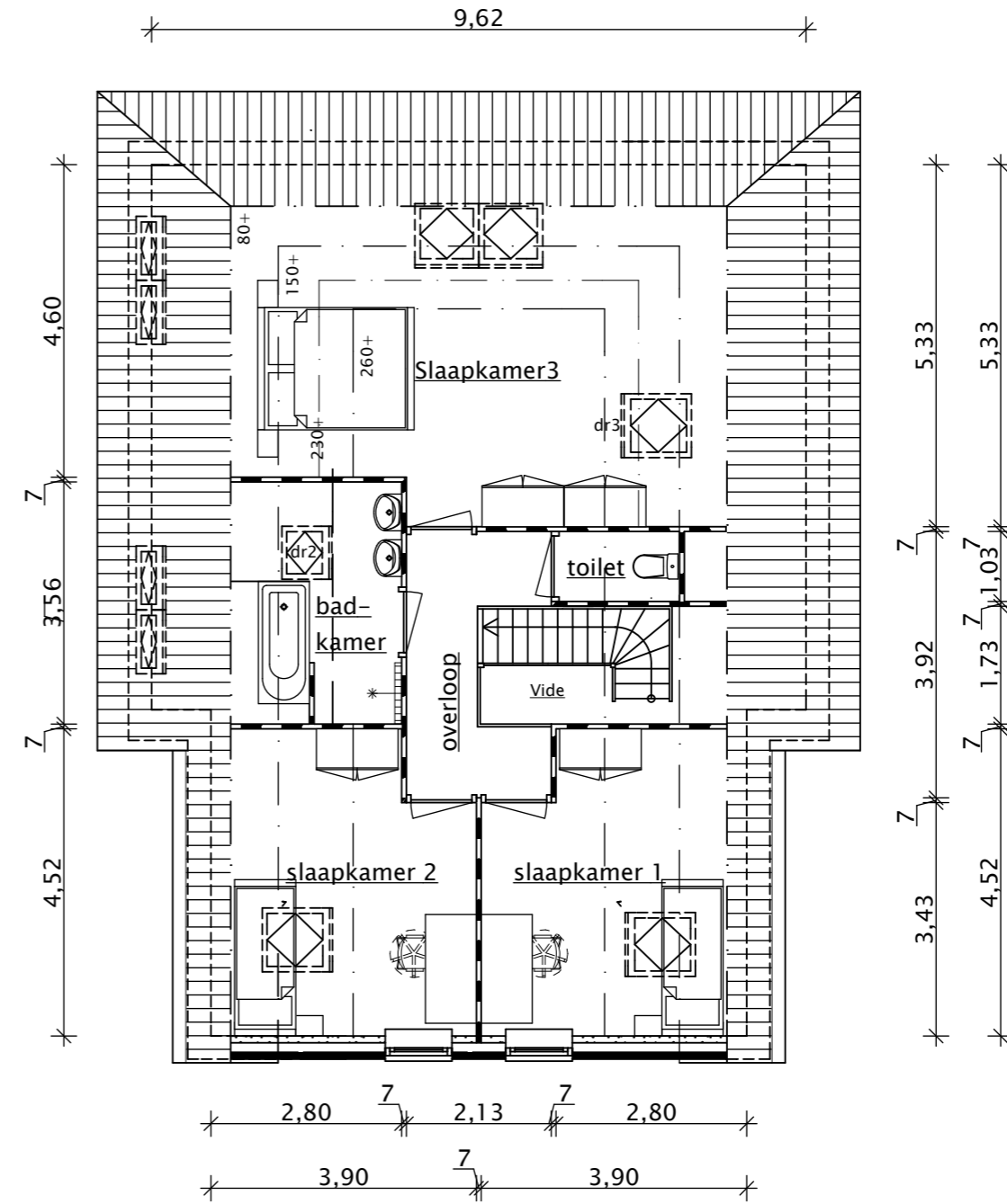
plattegrond Verdieping
