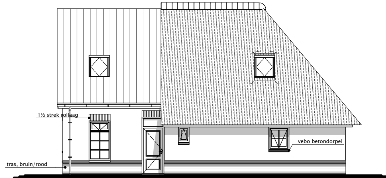
aanzicht Rechterzijgevel
