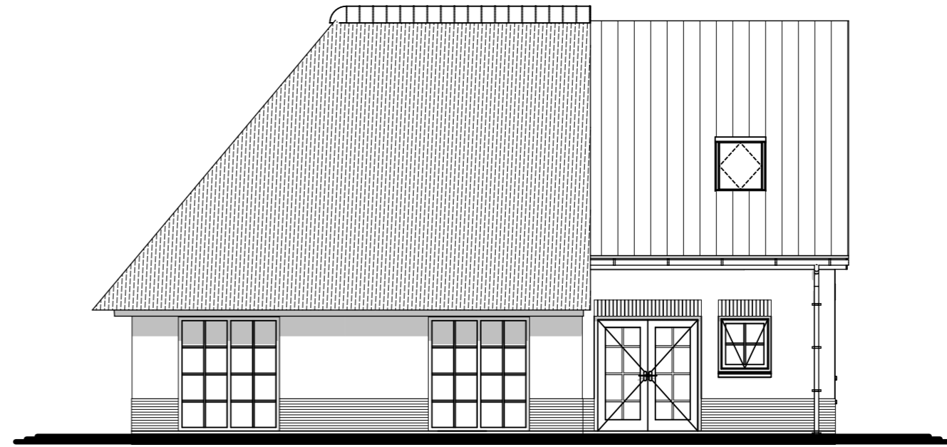
aanzicht Linkerzijgevel
