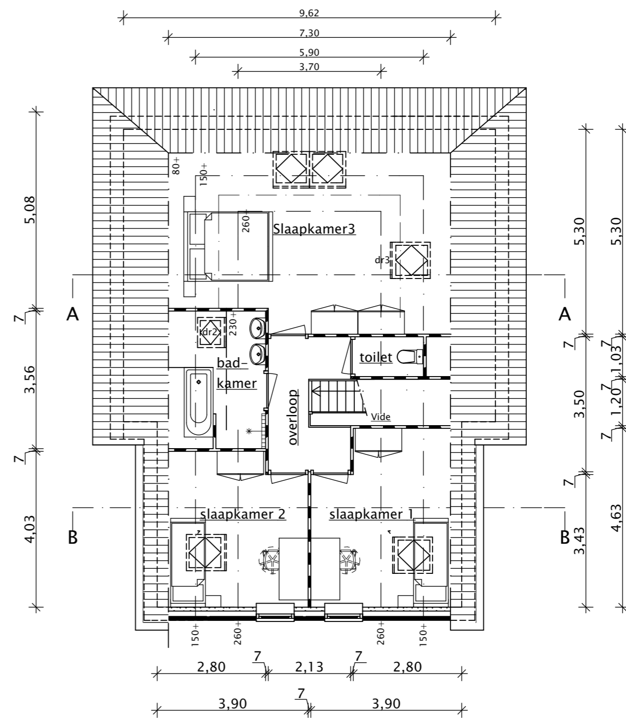
plattegrond VERDIEPING
