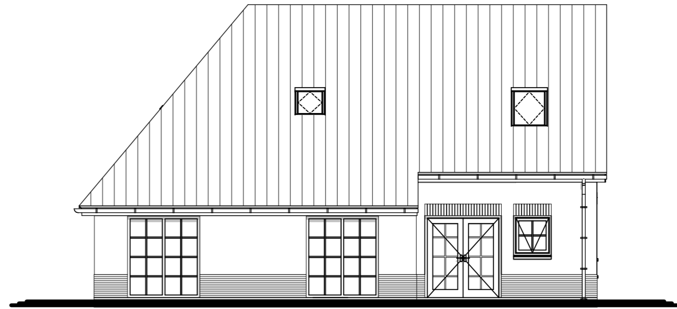
aanzicht Linkerzijgevel
