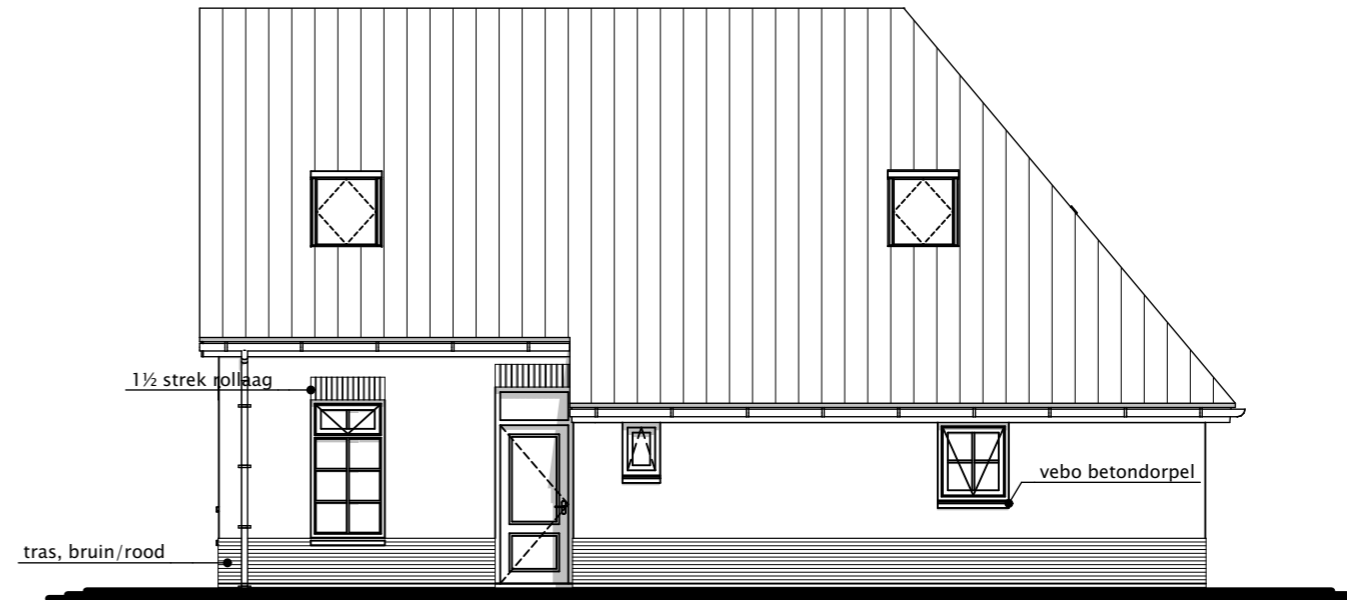
aanzicht Rechterzijgevel
