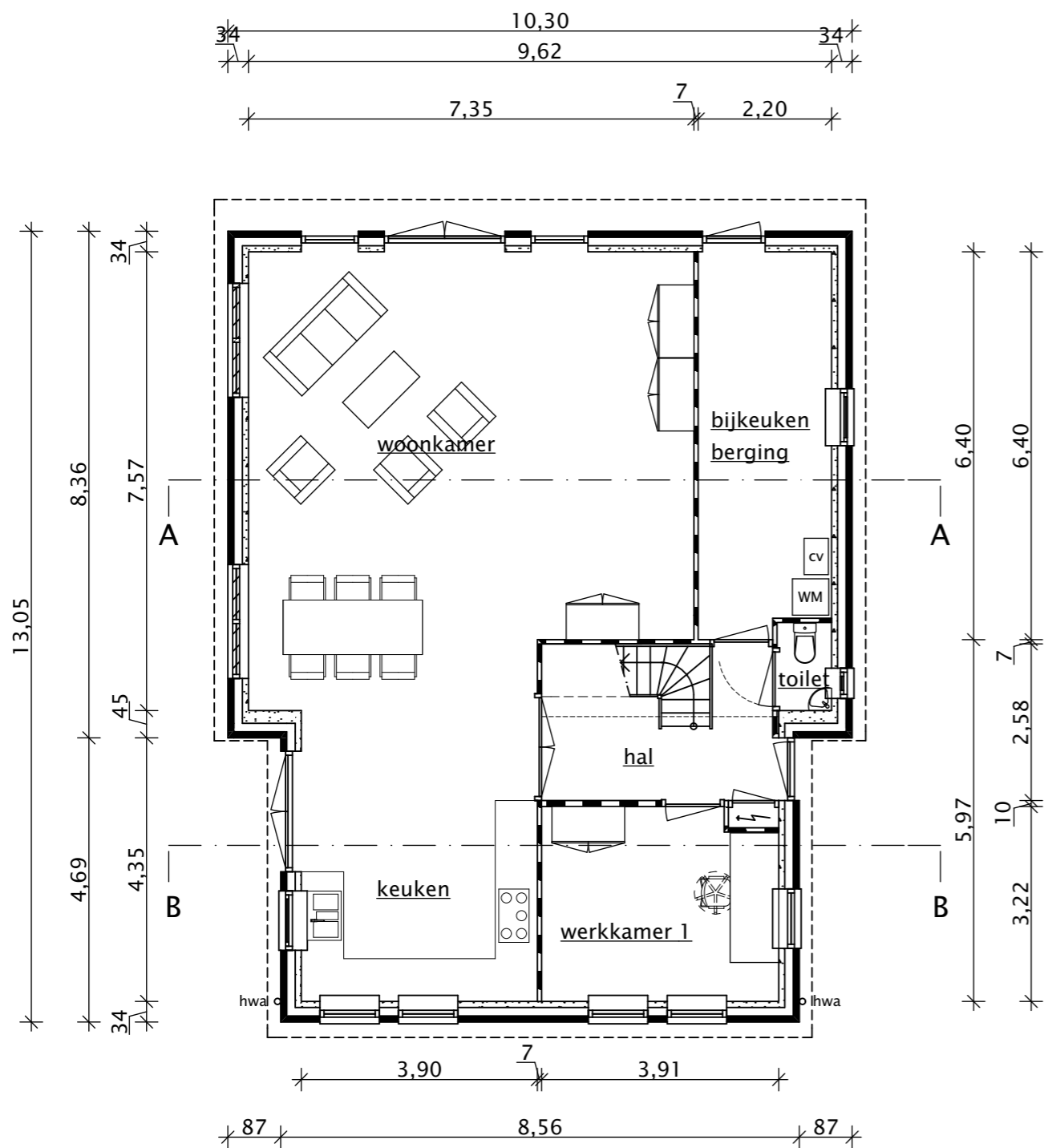
plattegrond BEGANEGROND
