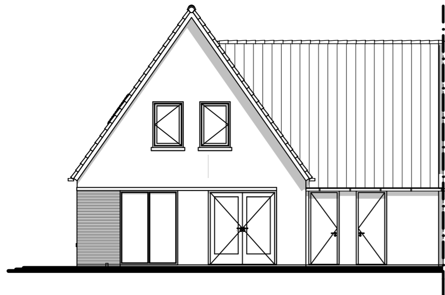
aanzicht Achtergevel
