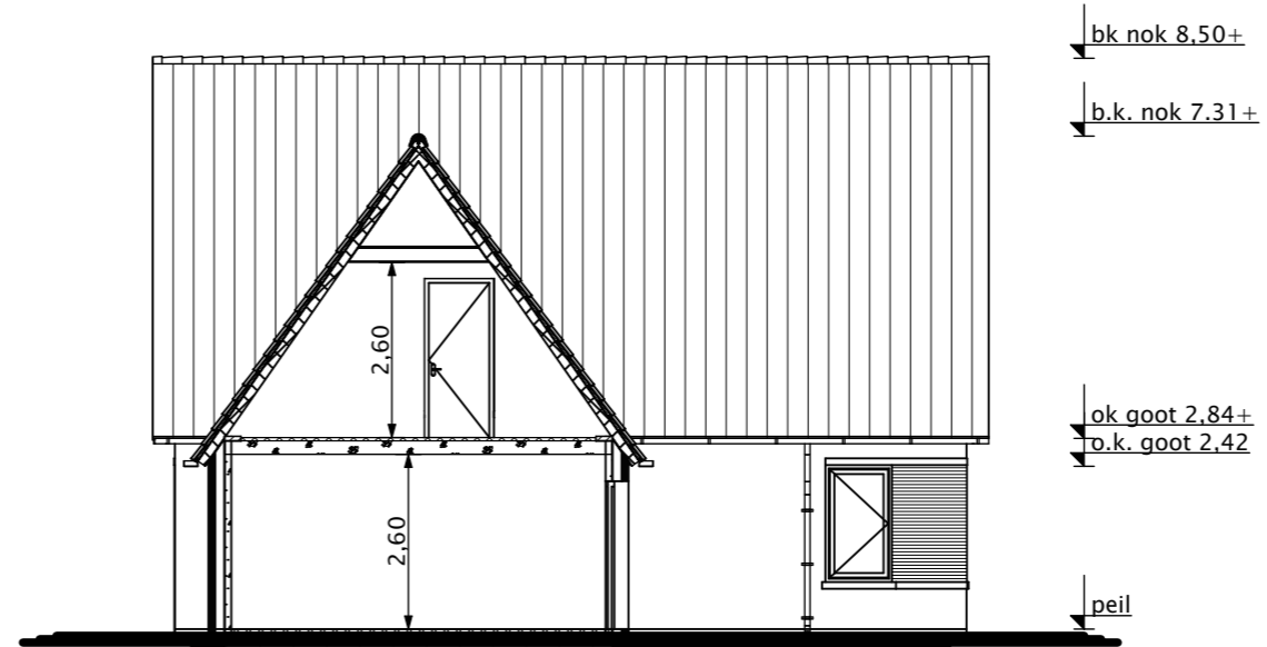
aanzicht Linkergevel
